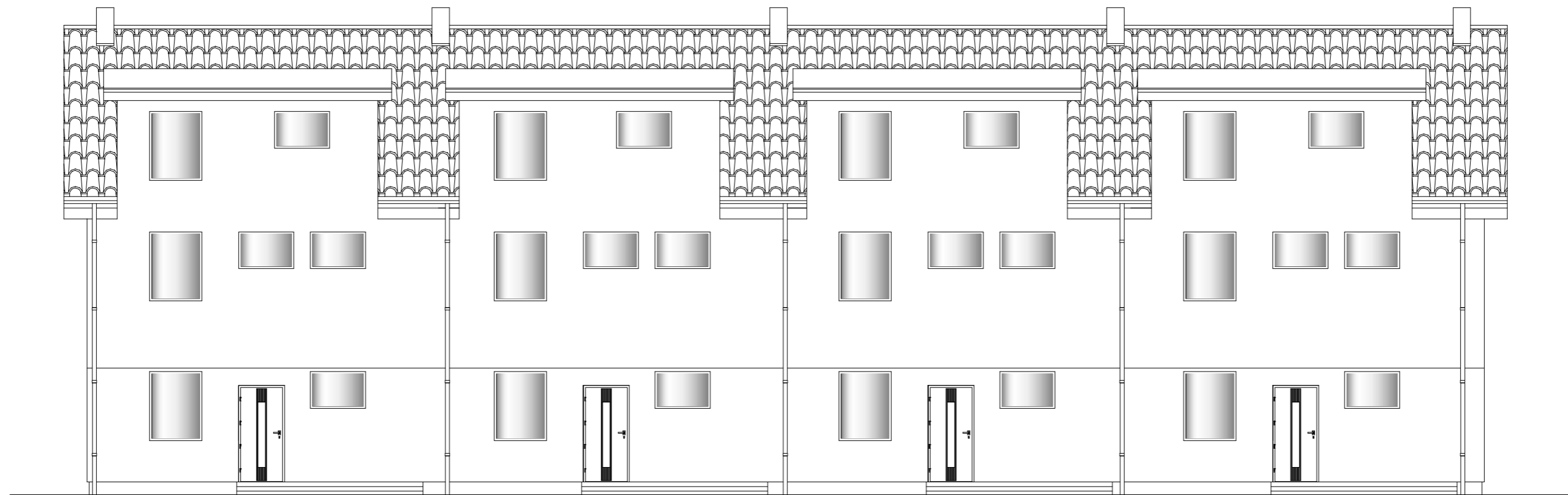
ELEWACJA WSCHODNIA 1:100
