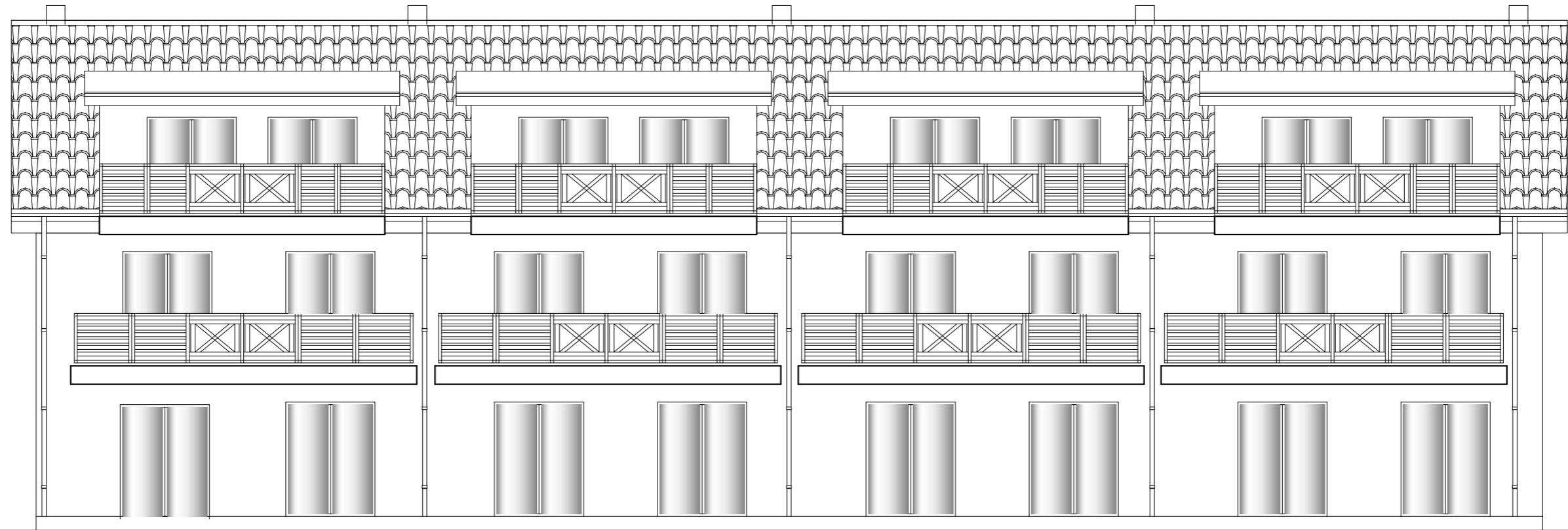
ELEWACJA ZACHODNIA 1:100
